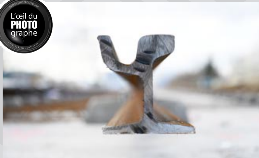
Profil d'un rail du futur tramway T9
